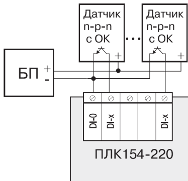
Рисунок Б.5 - Схема подключения к ПЛК154 дискретных датчиков с полупроводниковым выходным каскадом
