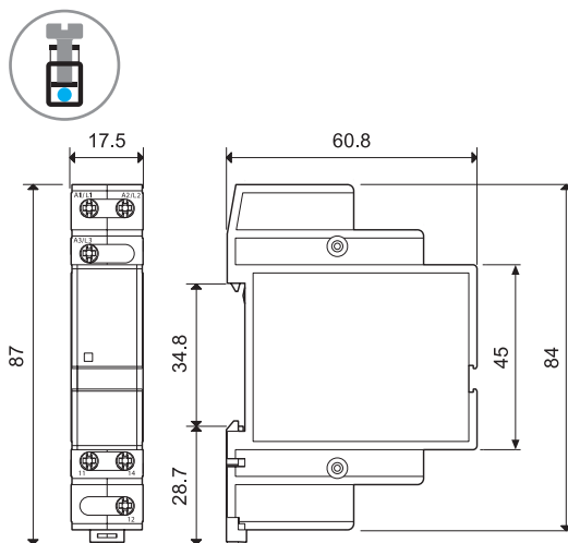
70.61 Винтовой клеммы
